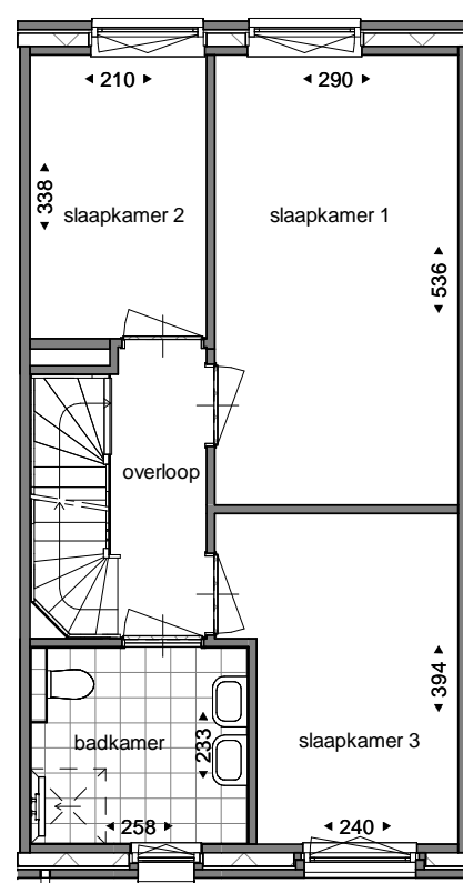
eerste verdieping
