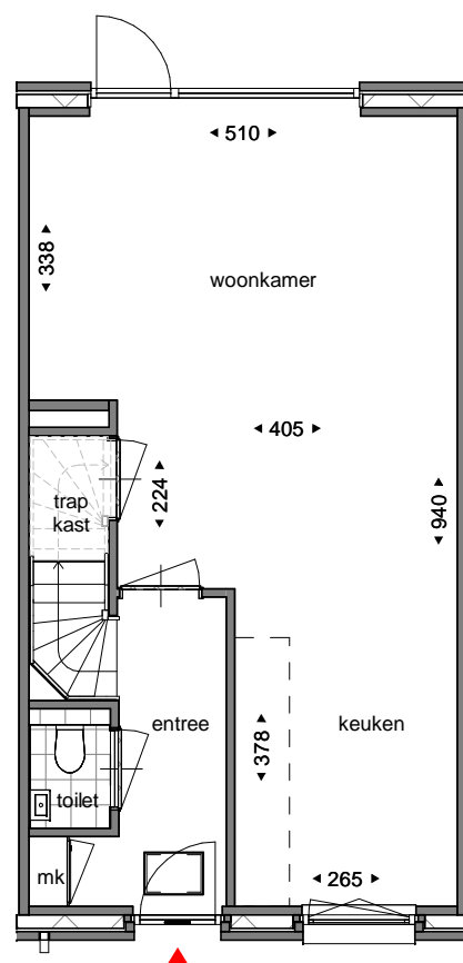
begane grond
